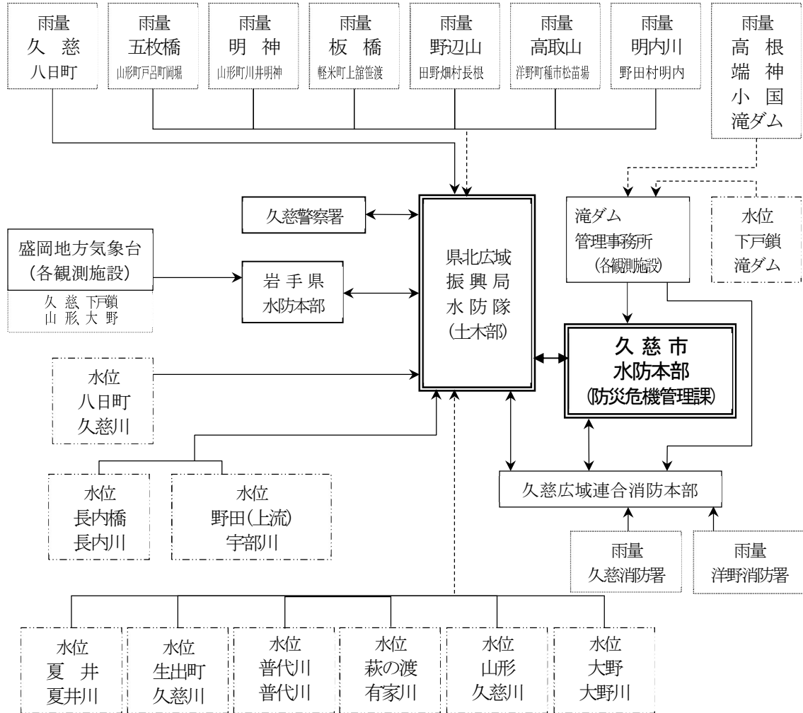
別表6 - 2(4) - 2 雨量、水位観測所及び関係機関の連絡系統図
