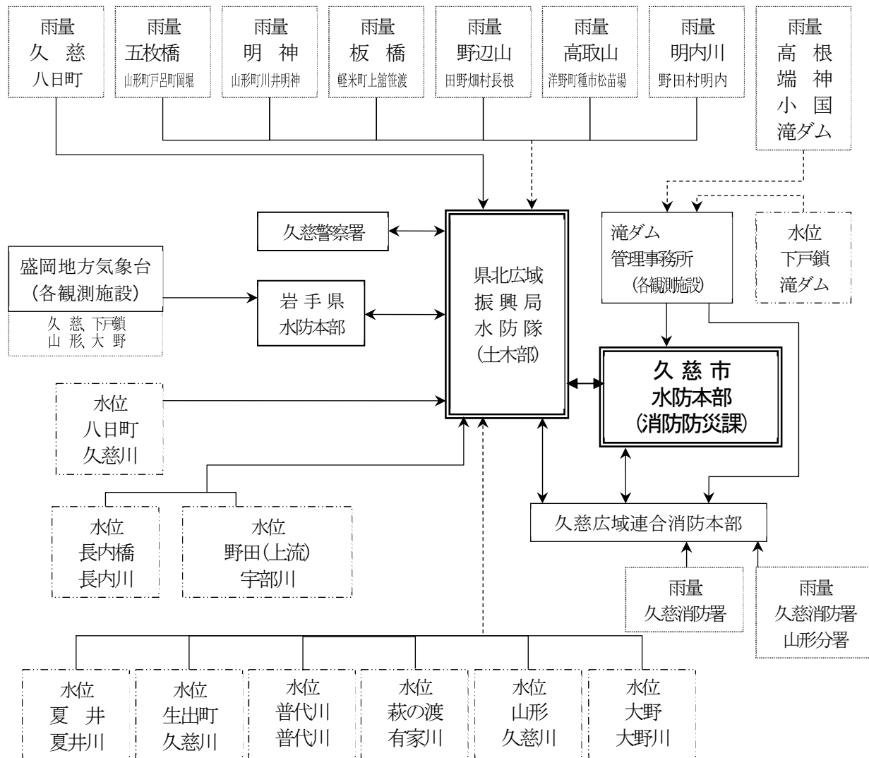
別表6 - 2(4) - 2 雨量、水位観測所及び関係機関の連絡系統図
