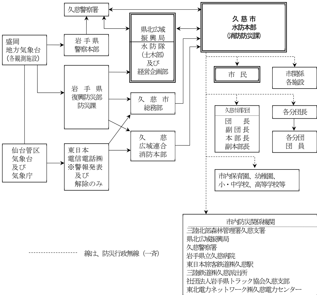
別表9 - 2 気象広報伝達系統図
